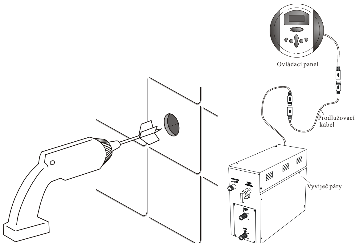
Obr.2 Vrtání otvoru a schéma propojení
