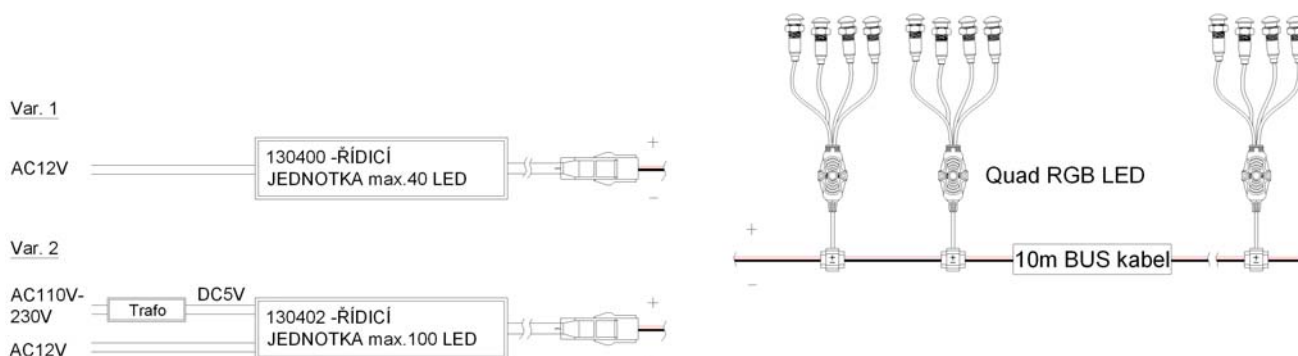
Ukázka napojení klipu na řídicí vodič
